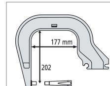
Bras C8 8 bar/550 daN
