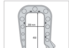
Bras C4 8 bar/550 daN
