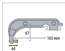
Bras C12 8 bar/550 daN
