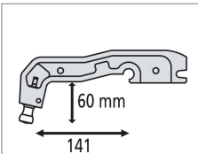
Bras C6 8 bar/300 daN
