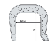
Bras C7 8 bar/550 daN
